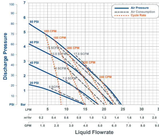
PXHSD030
