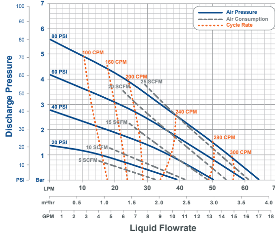
PXHSD060
