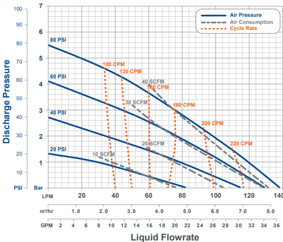
PXH140
